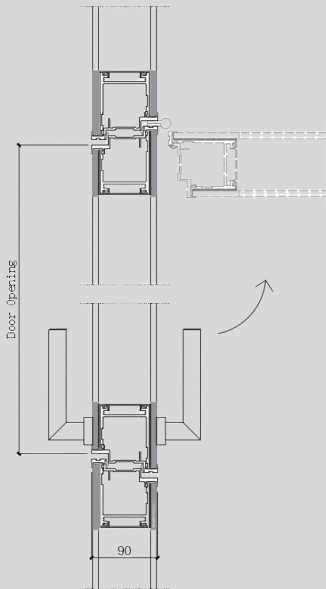
Door Detail
