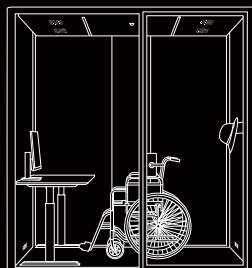
W2200*D1770*H2200mm
